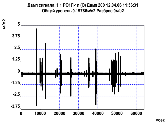
Рис. 2. Временной сигнал подшипника с одиночным дефектом (длительность 64 сек)
