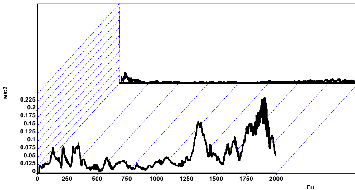
Рис. 3. Окно сравнения спектров (ближний спектр получен на подшипнике с дефектом, дальний – на бездефектном подшипнике)
